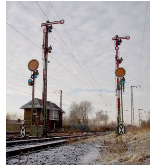
Formsignale Eisenbahn
